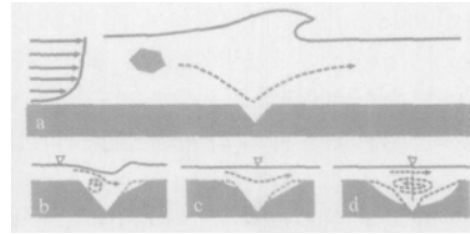
图 7 三角坑成因及发育过程示意图 Fig. 7 Schematic illustration for development of a triangular pit
